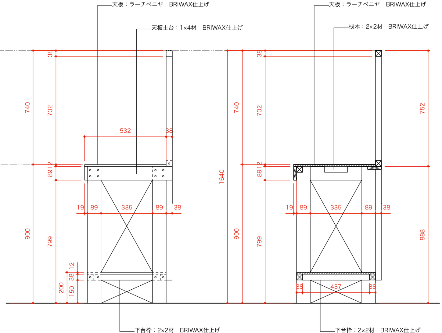
■断面図
